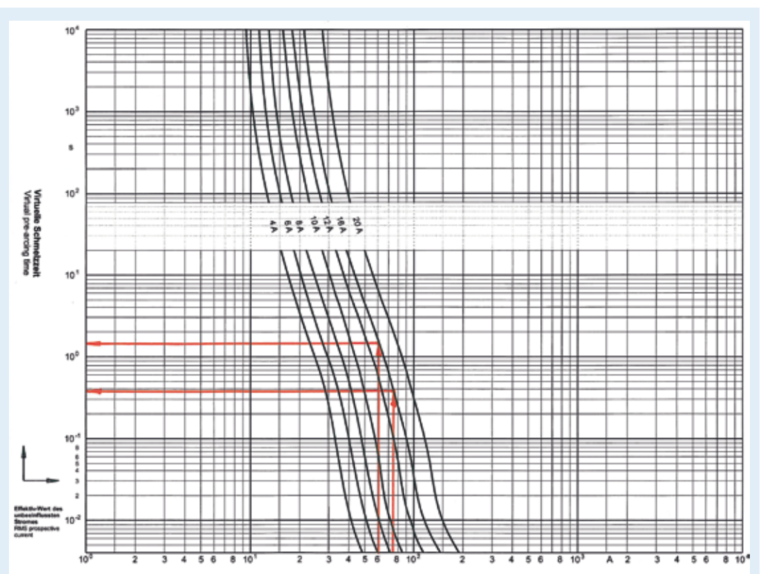
Bild 3: Zeit/Strom-Kennlinien der gewählten PV-Fuse
